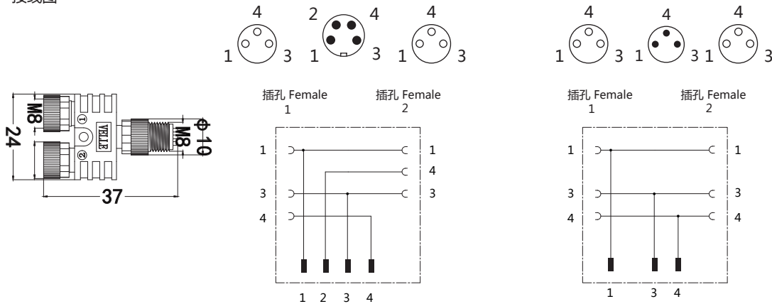
接线图
