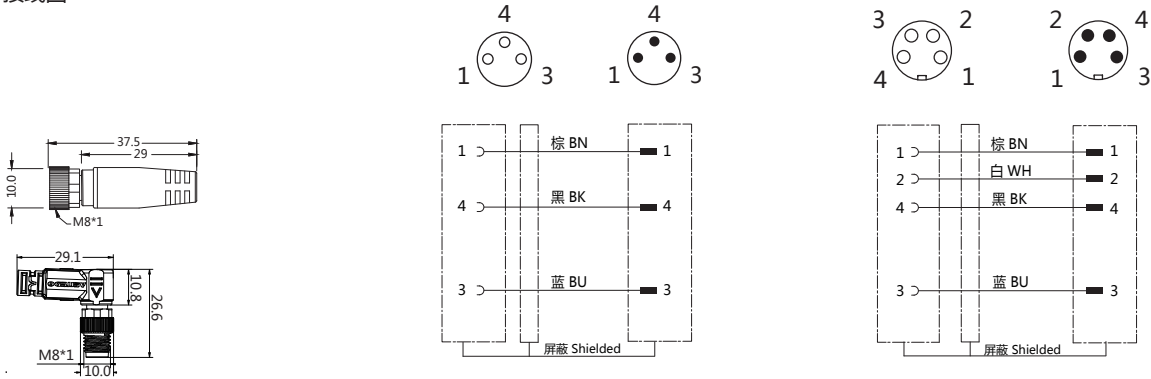
接线图
