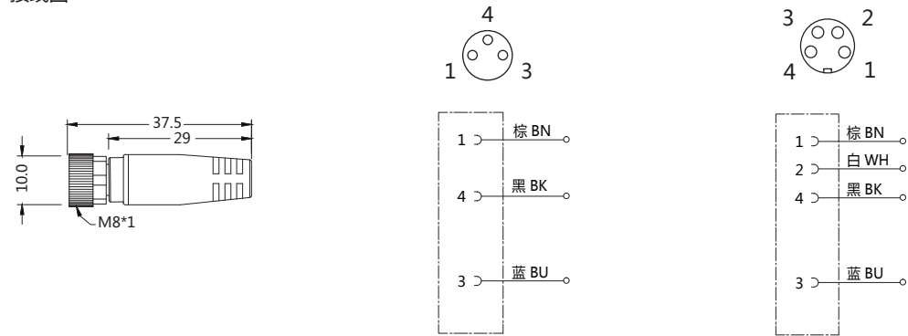
接线图
