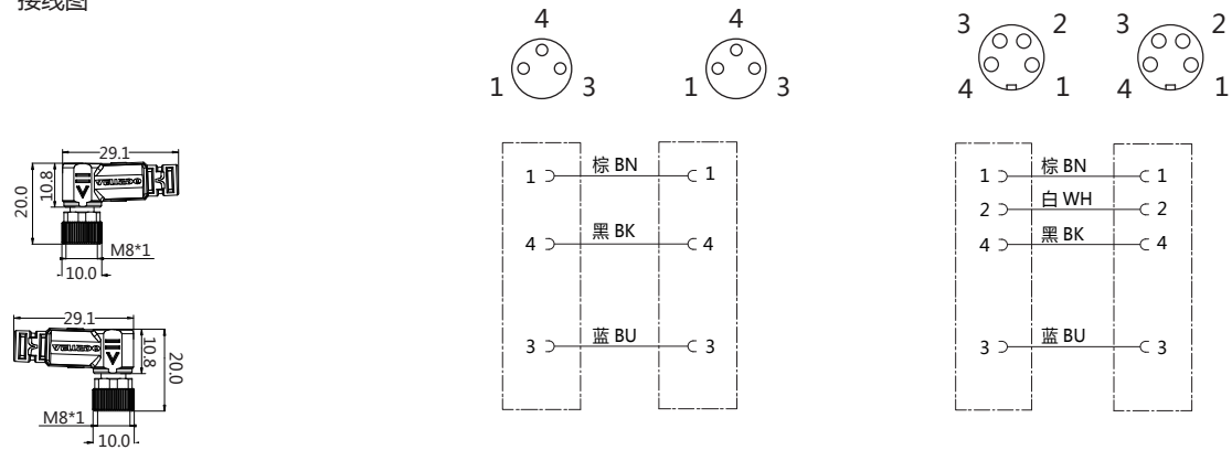
接线图
