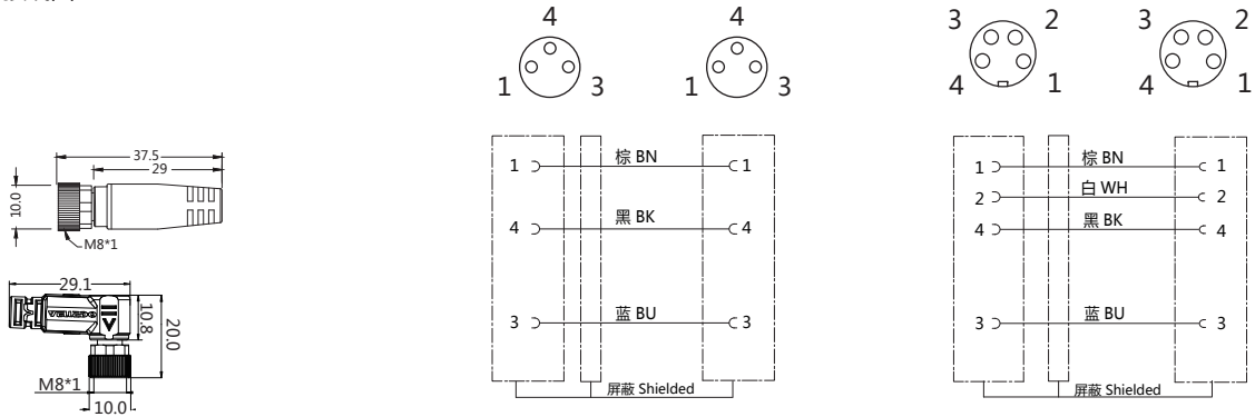
接线图
