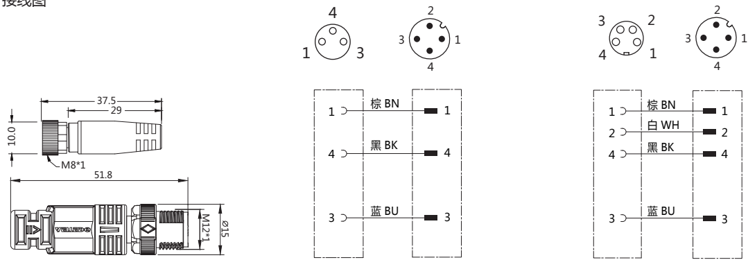
接线图
