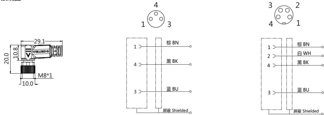
接线图
