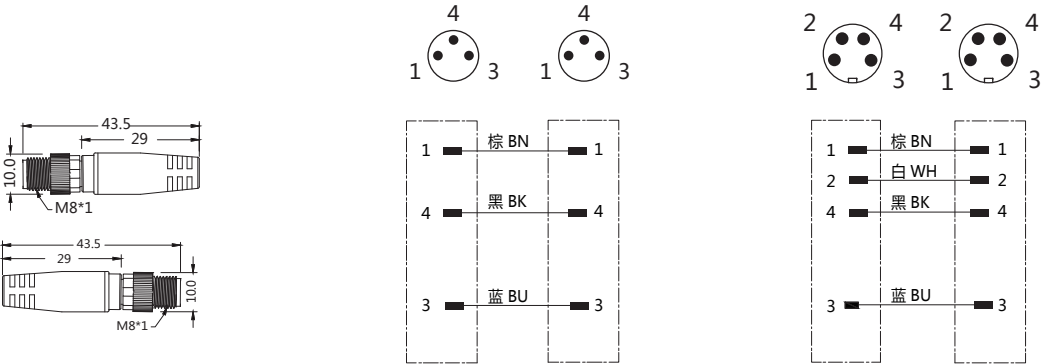
接线图
