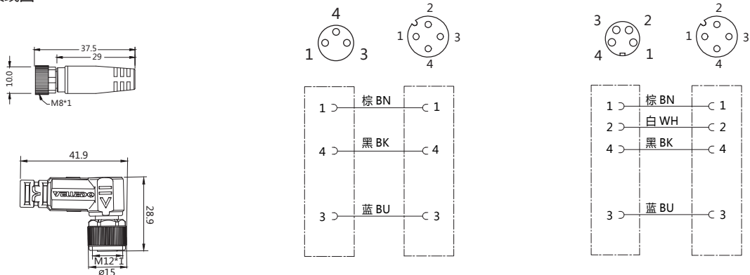
接线图
