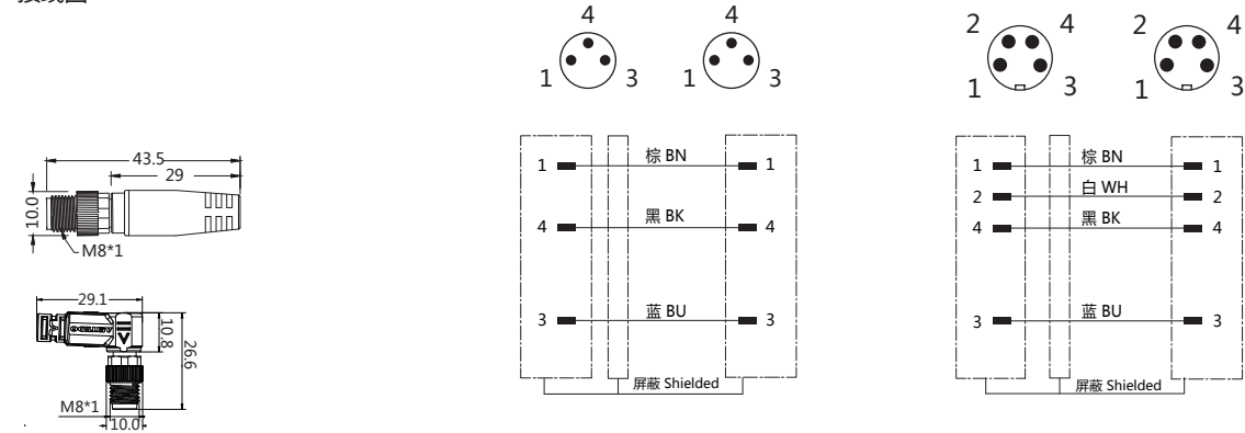
接线图
