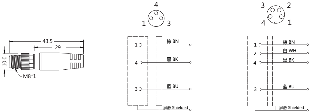
接线图
