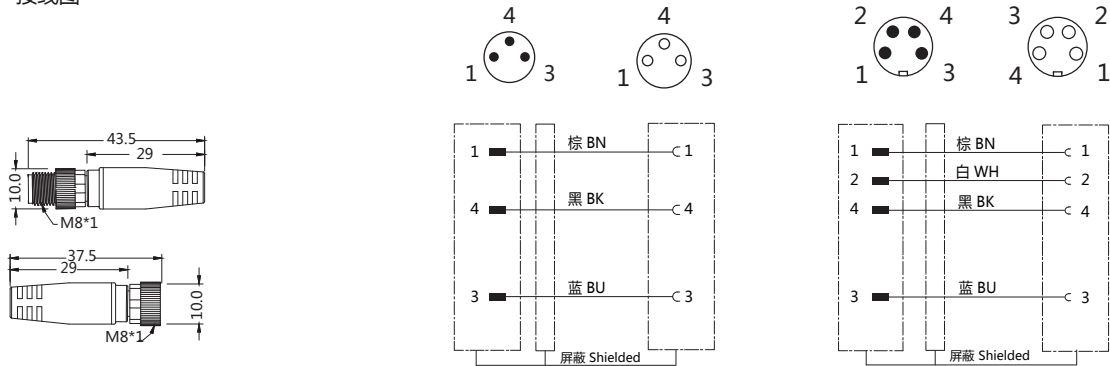
接线图
