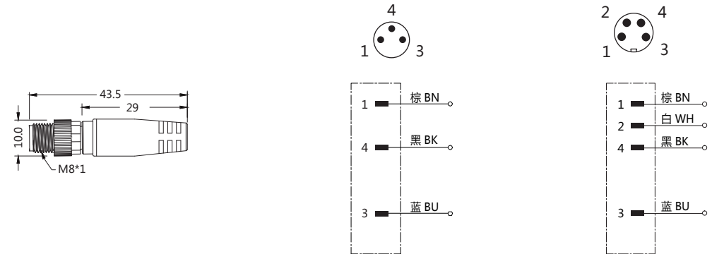
接线图
