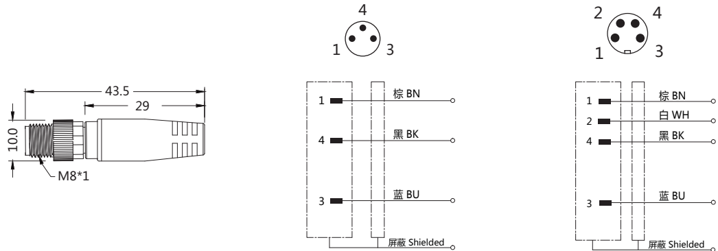
接线图
