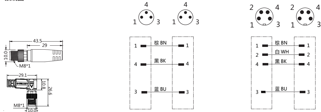
接线图
