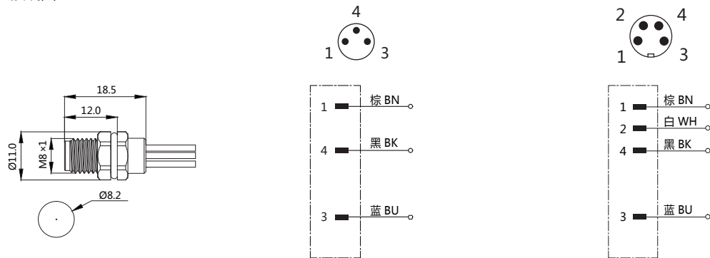
接线图
