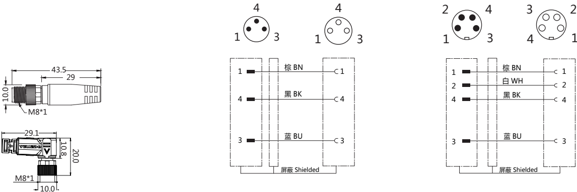
接线图
