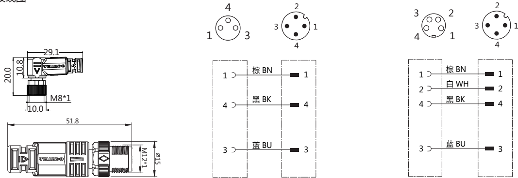
接线图
