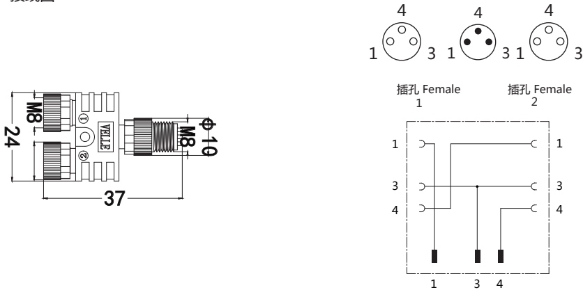
接线图
