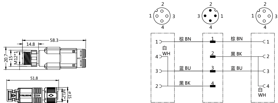
接线图
