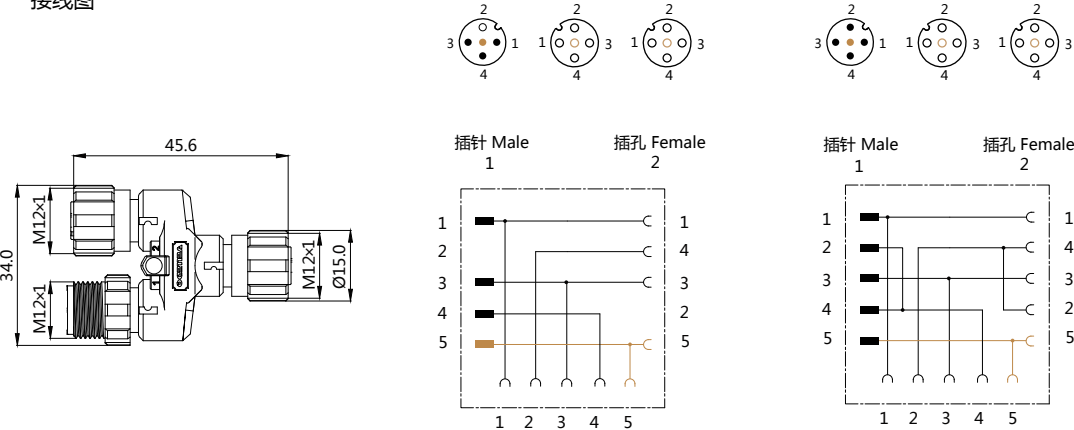
接线图
