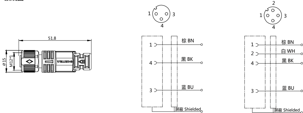
接线图
