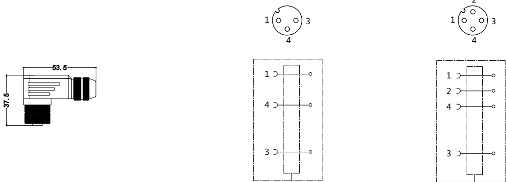
接线图
