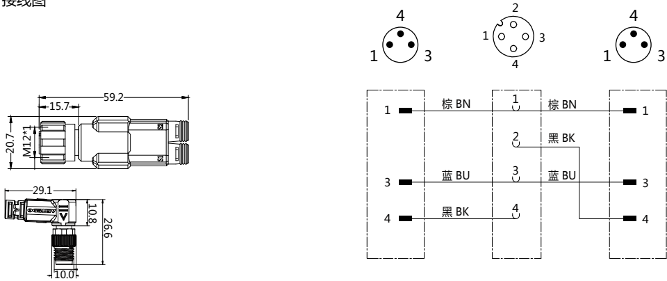
接线图
