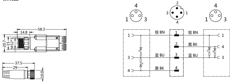
接线图
