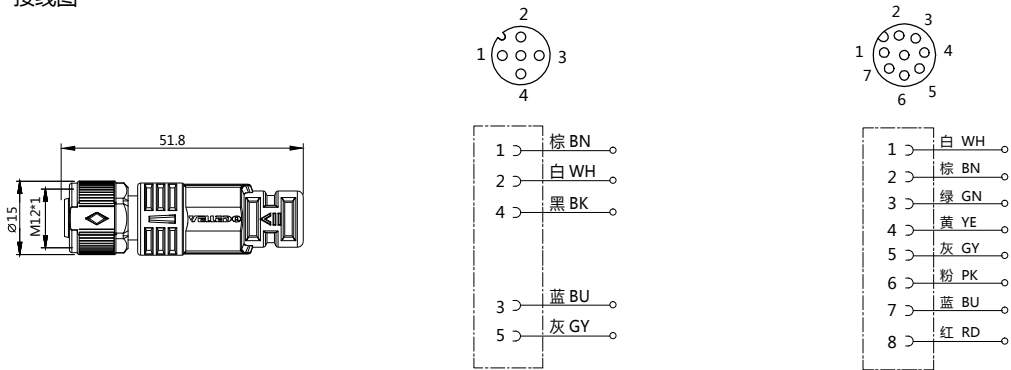
接线图
