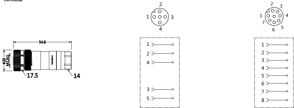
接线图
