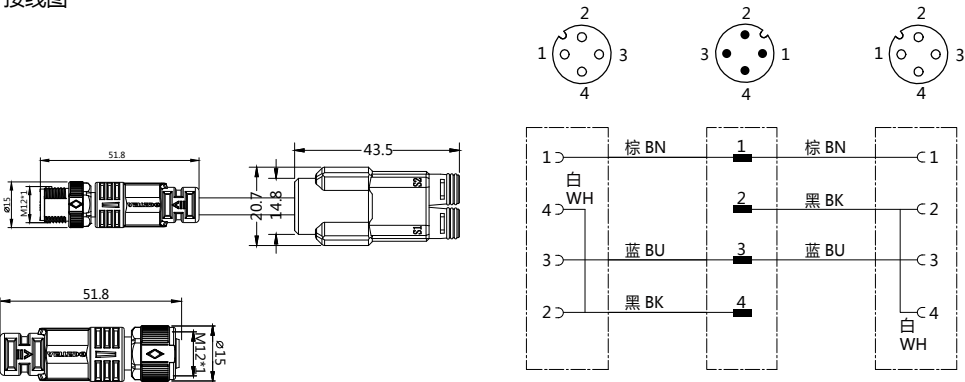
接线图
