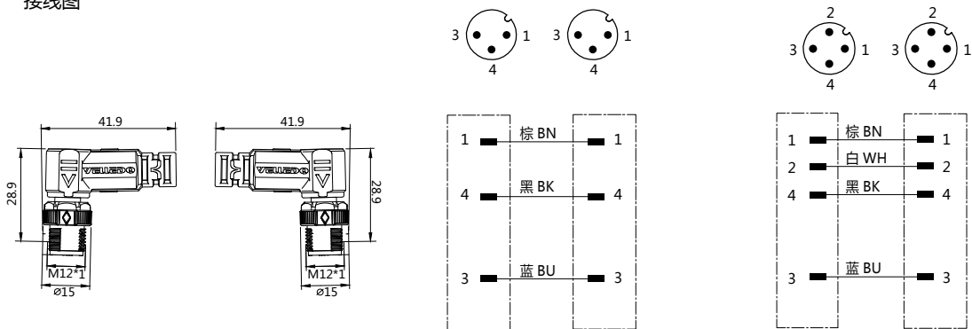
接线图
