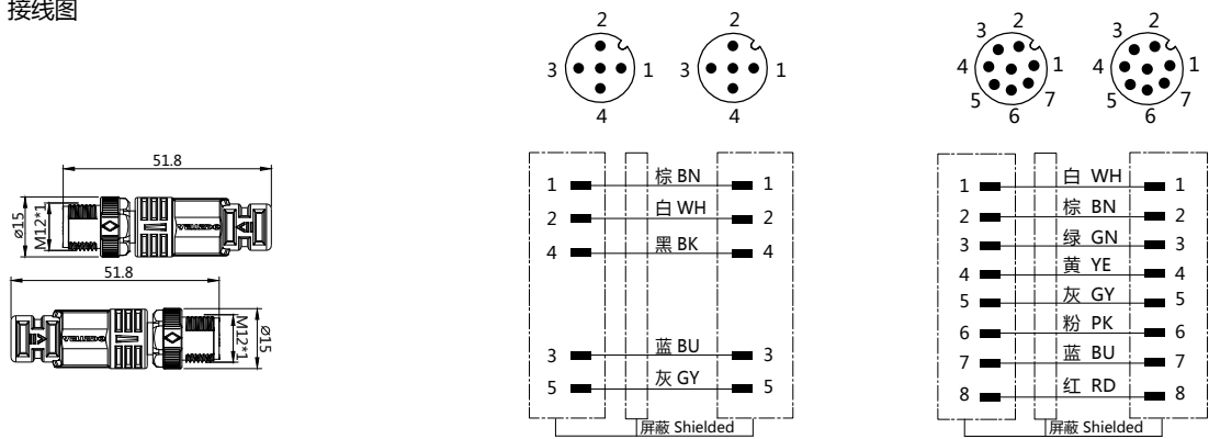
接线图
