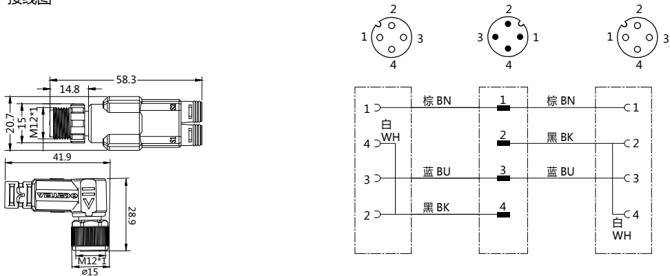
接线图
