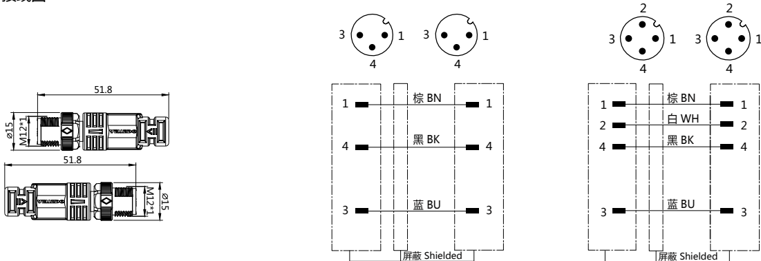
接线图
