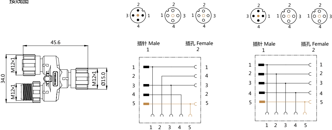
接线图
