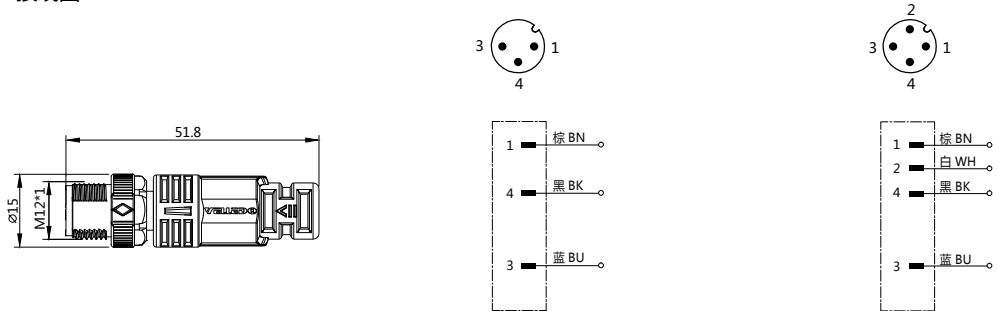
接线图
