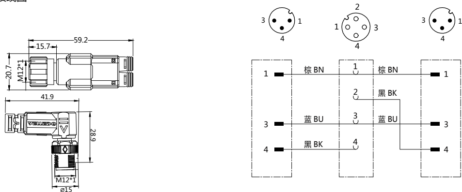
接线图
