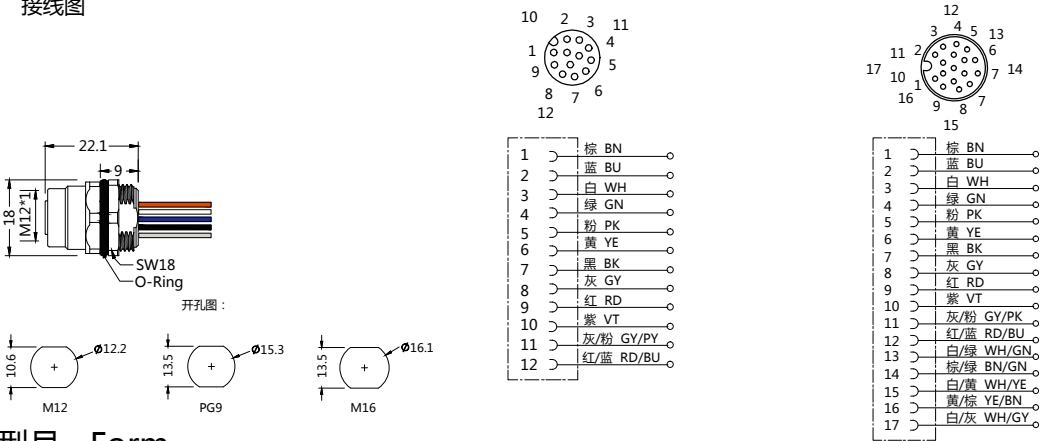
接线图
