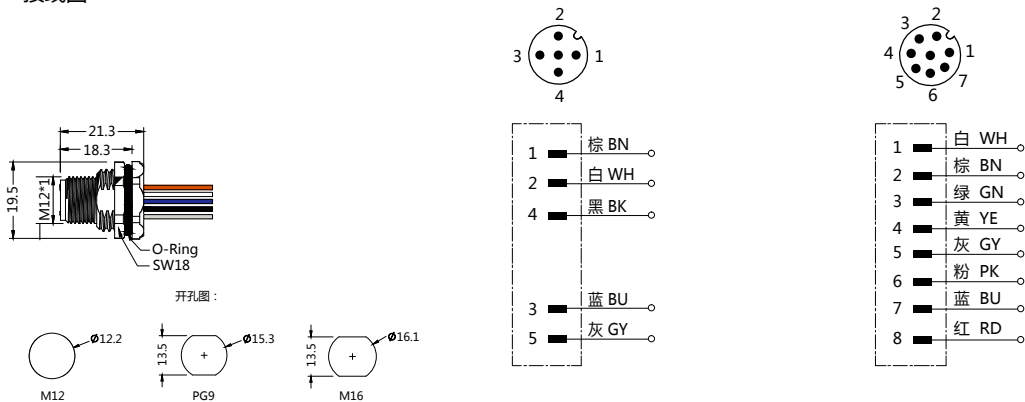
接线图
