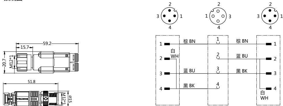
接线图
