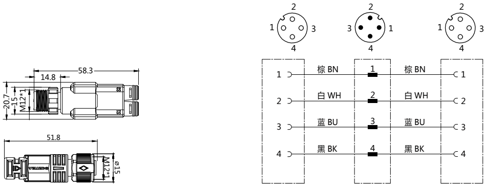
接线图
