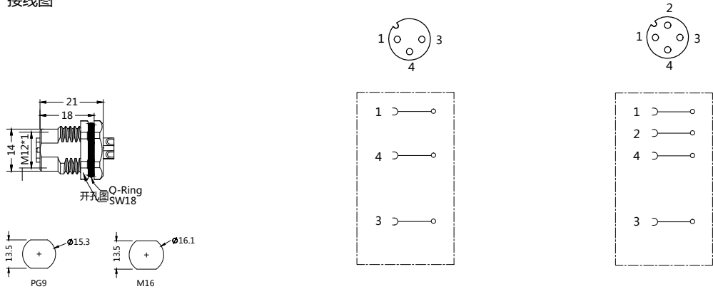
接线图
