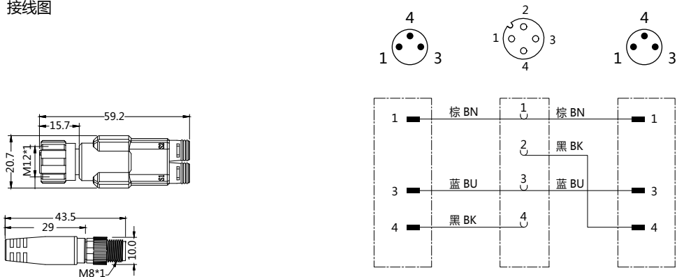
接线图
