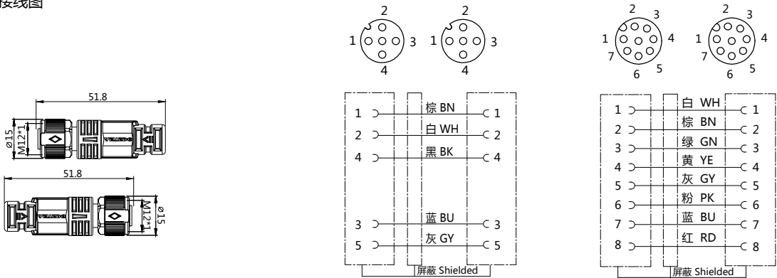
接线图
