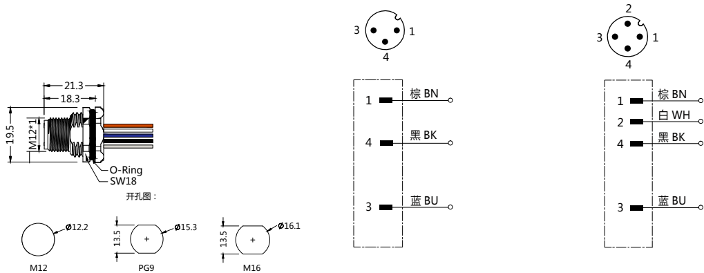
接线图
