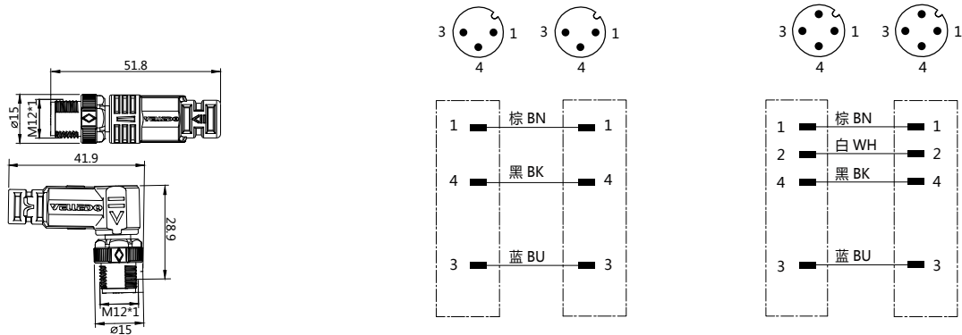
接线图
