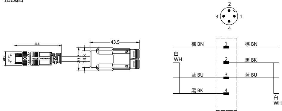
接线图
