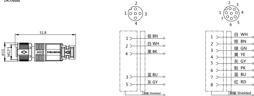
接线图
