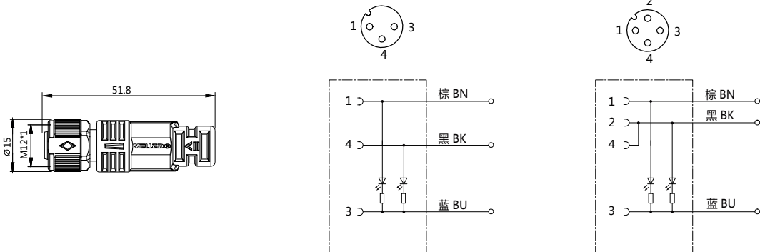
接线图
