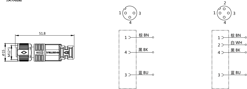
接线图
