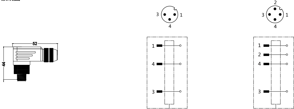
接线图
