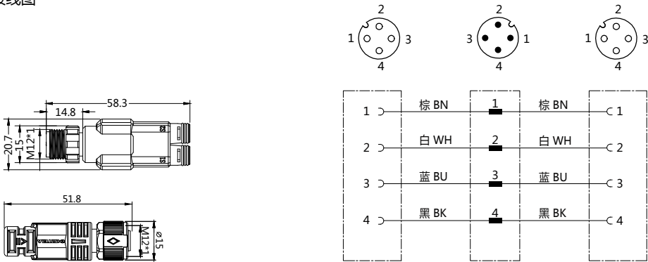
接线图
