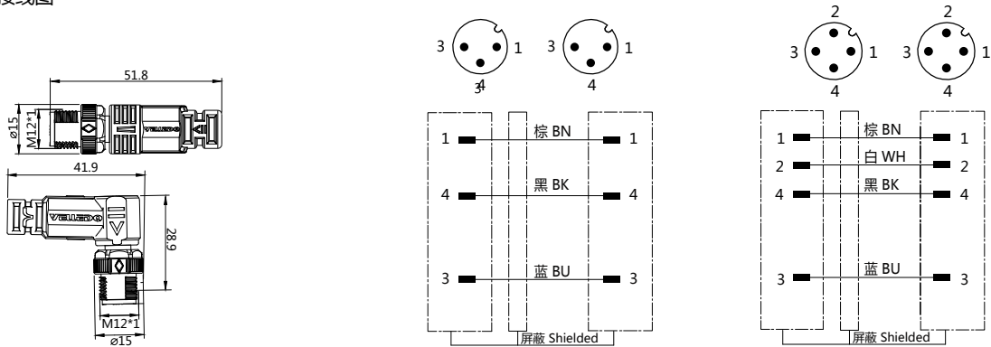
接线图
