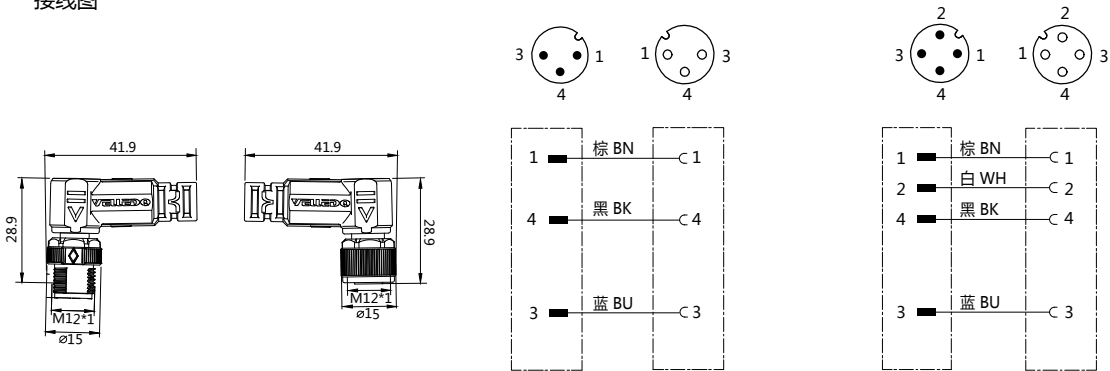
接线图
