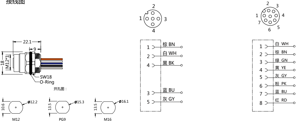
接线图
