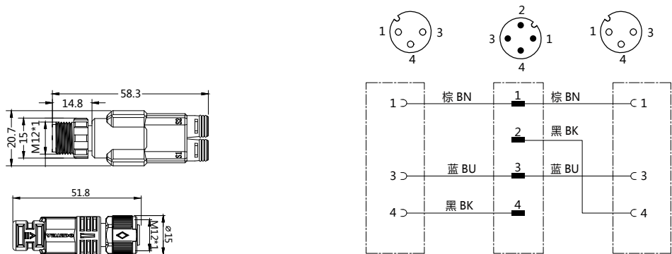
接线图
