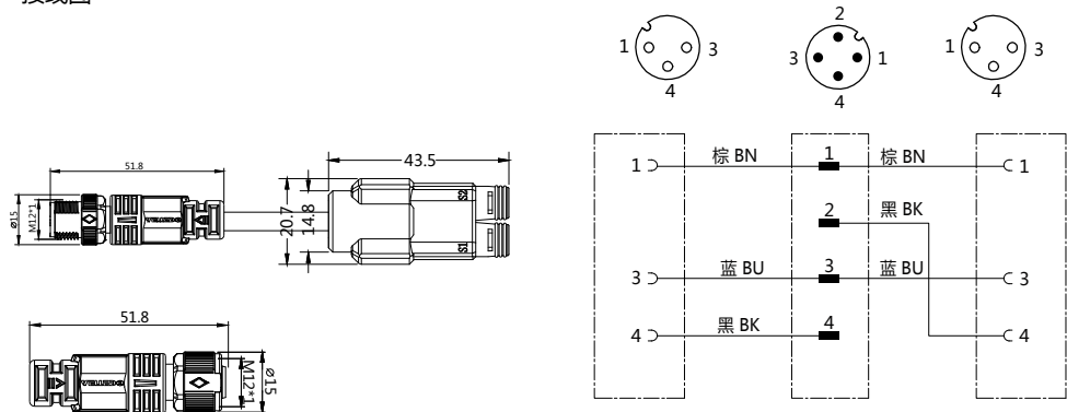
接线图
