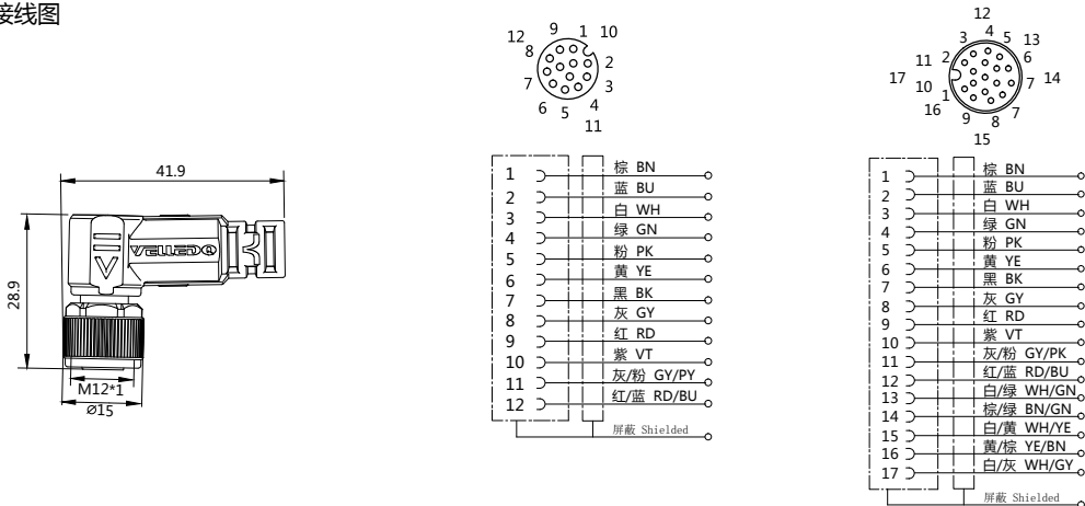
接线图
