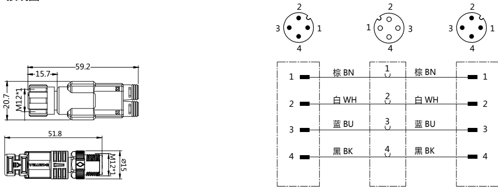
接线图
