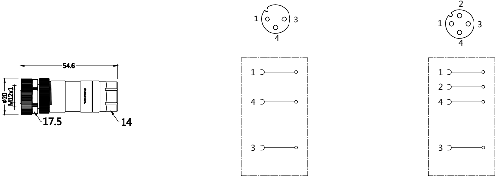
接线图
