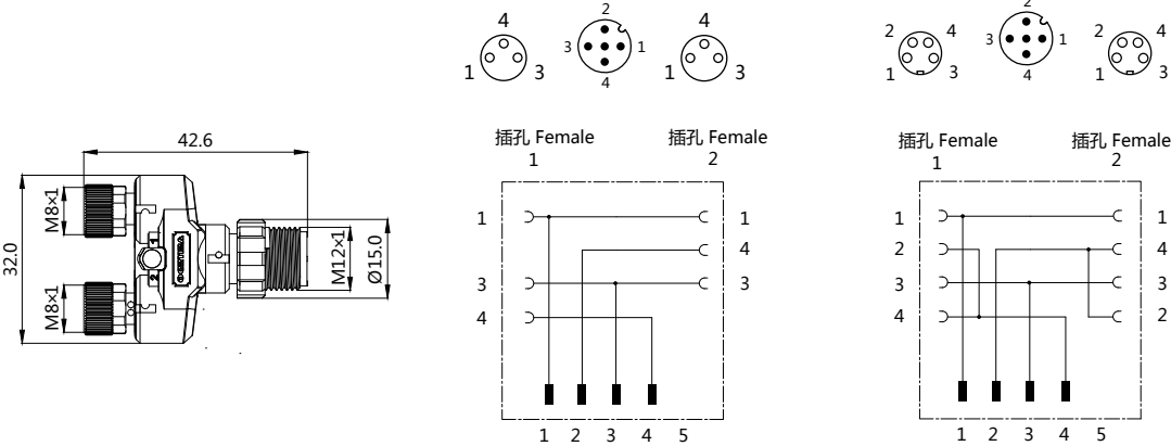
接线图
