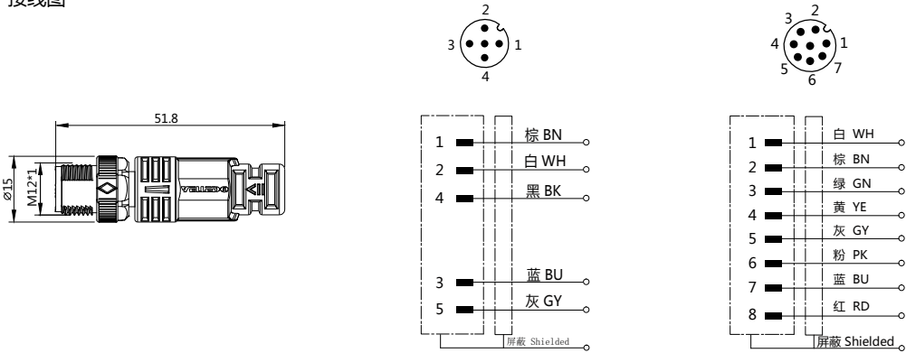
接线图
