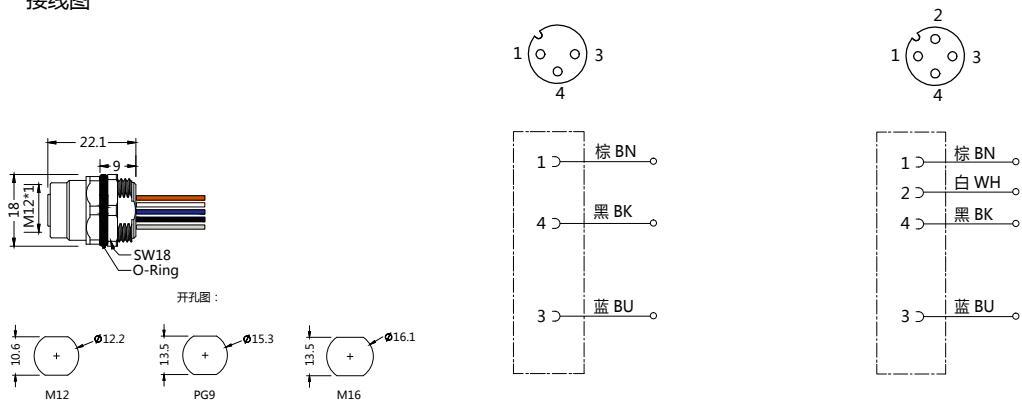
接线图
