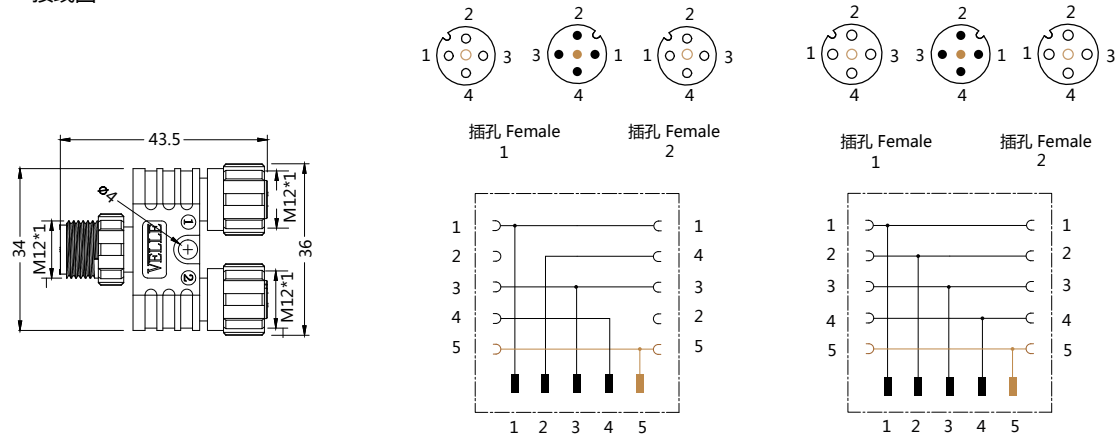
接线图
