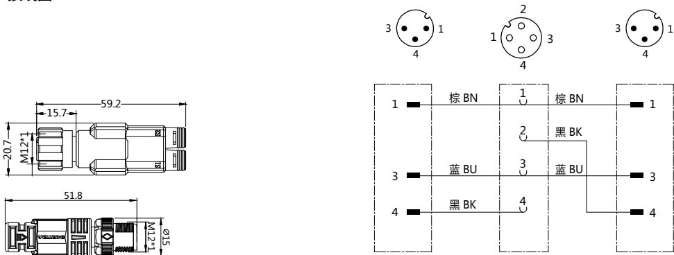
接线图
