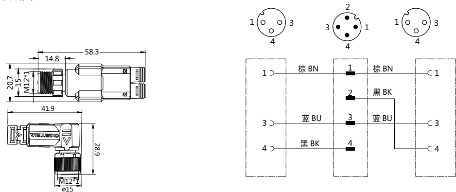
接线图
