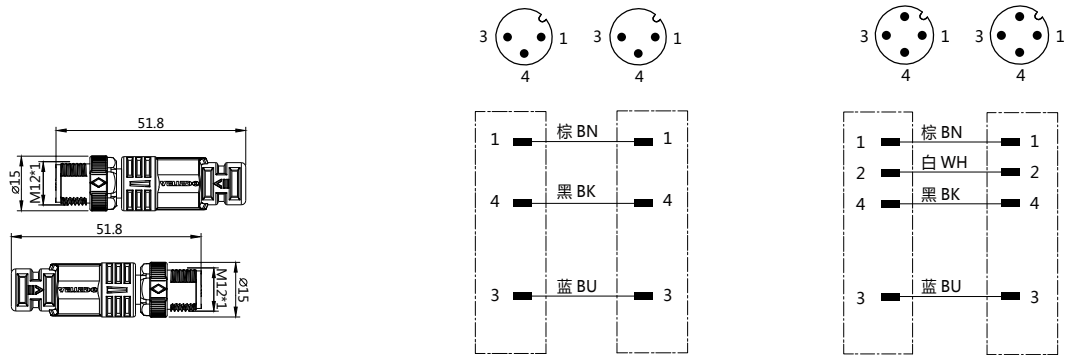
接线图
