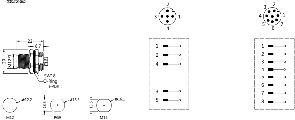
接线图
