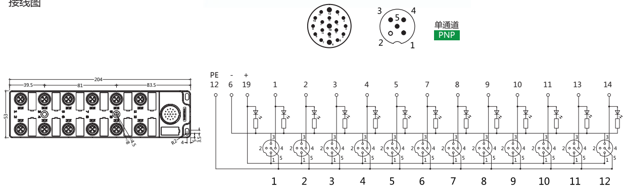
接线图
