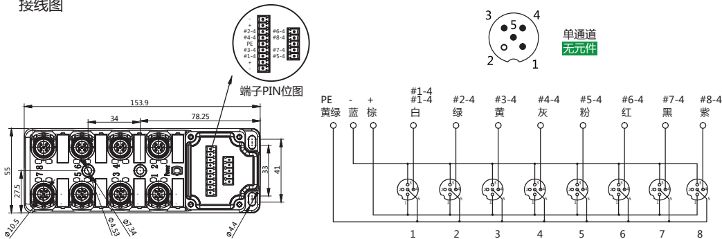
接线图
