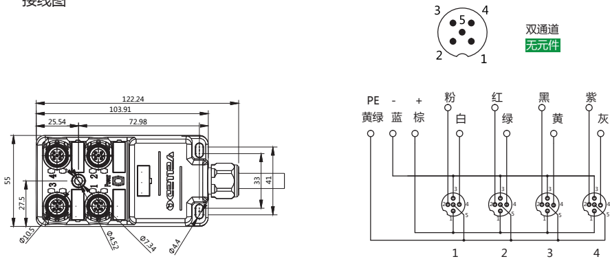
接线图
