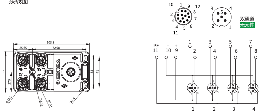
接线图
