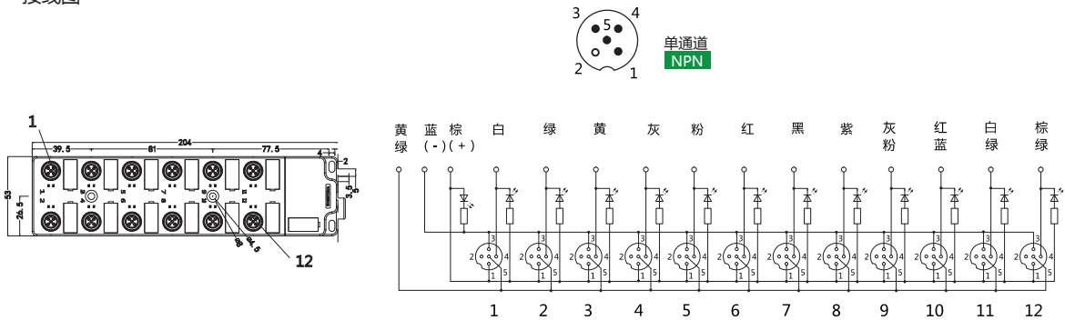
接线图
