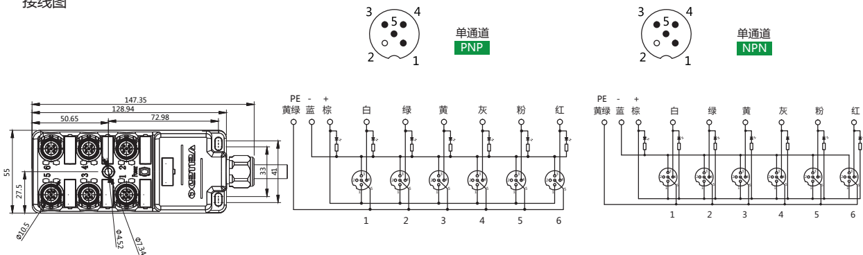
接线图
