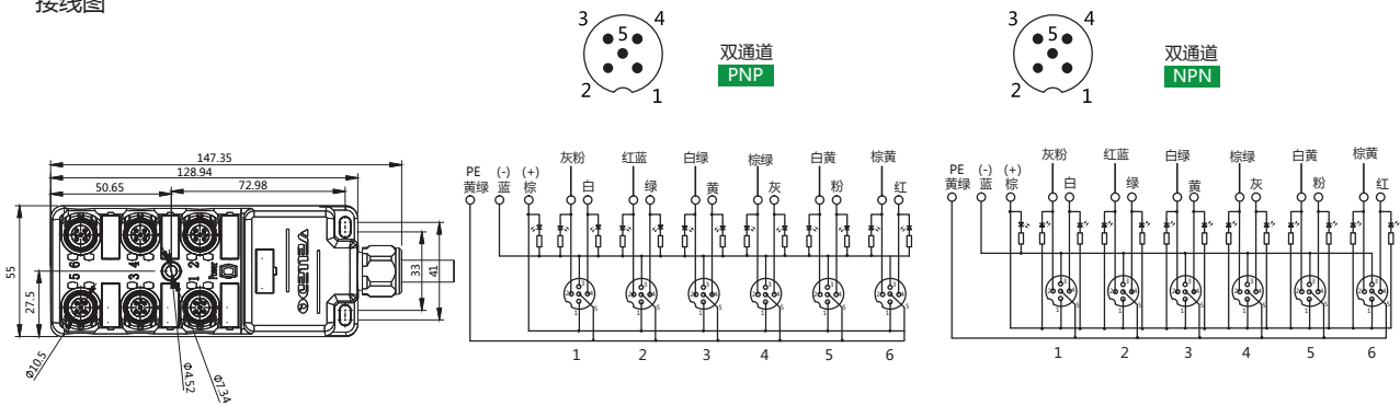
接线图
