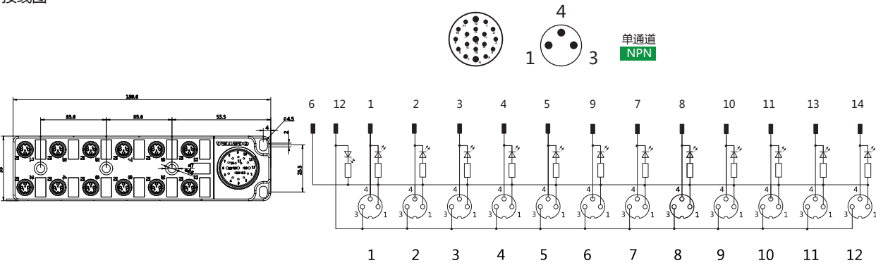
接线图
