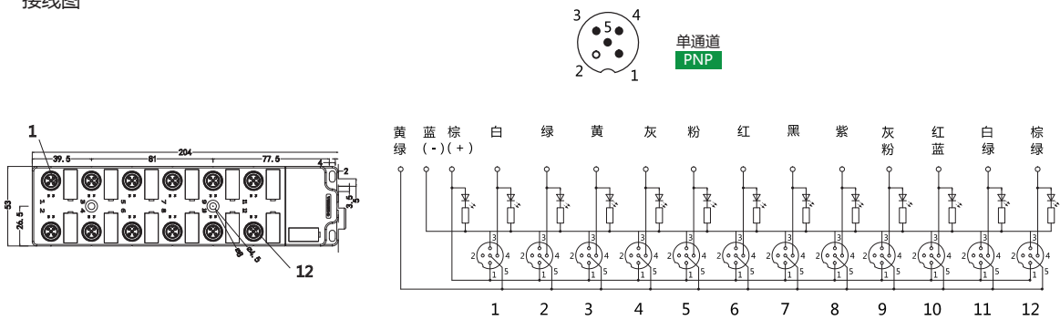
接线图
