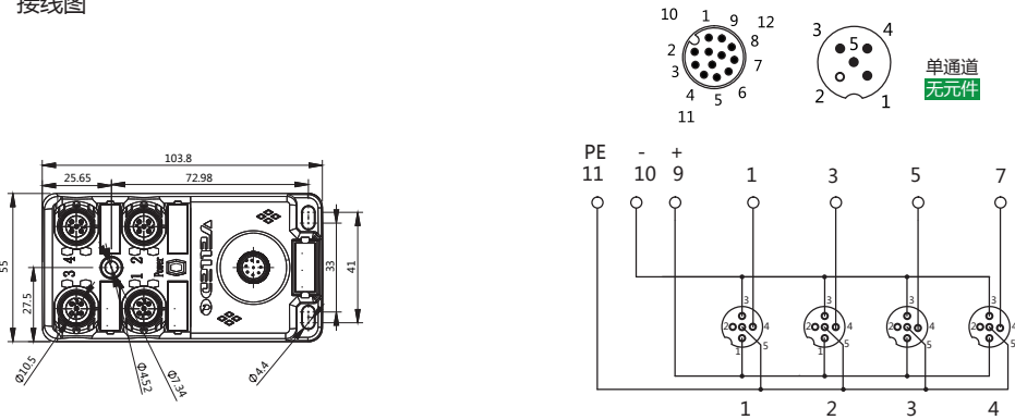
接线图
