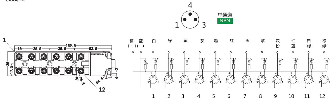
接线图
