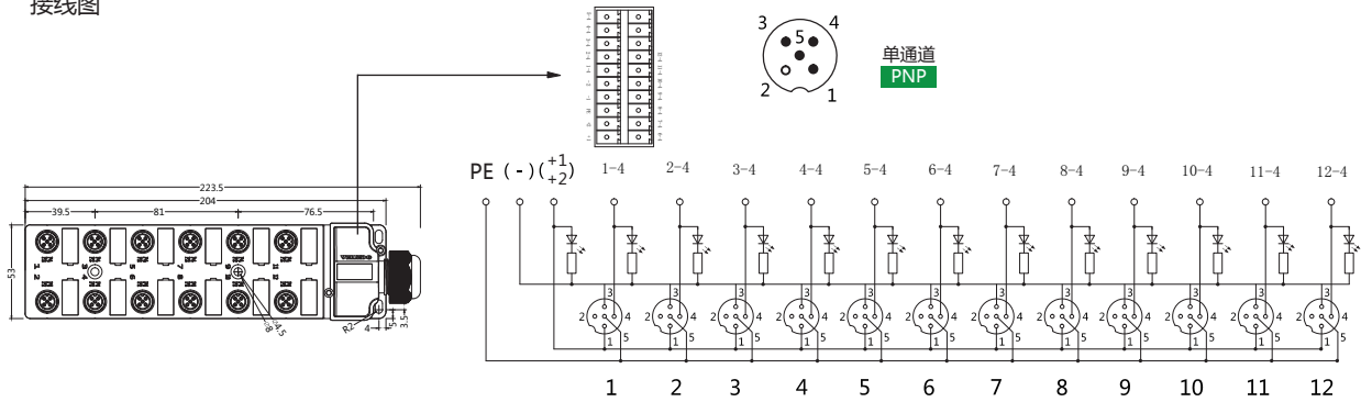
接线图
