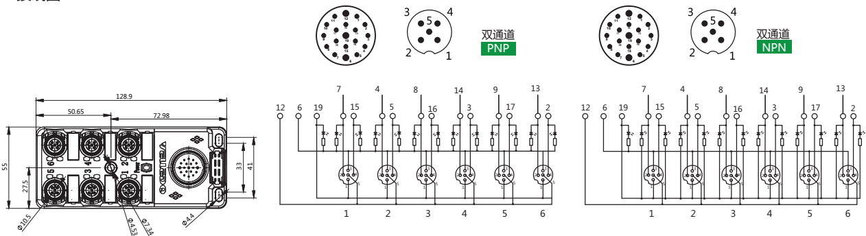
接线图
