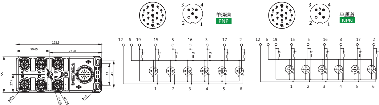
接线图
