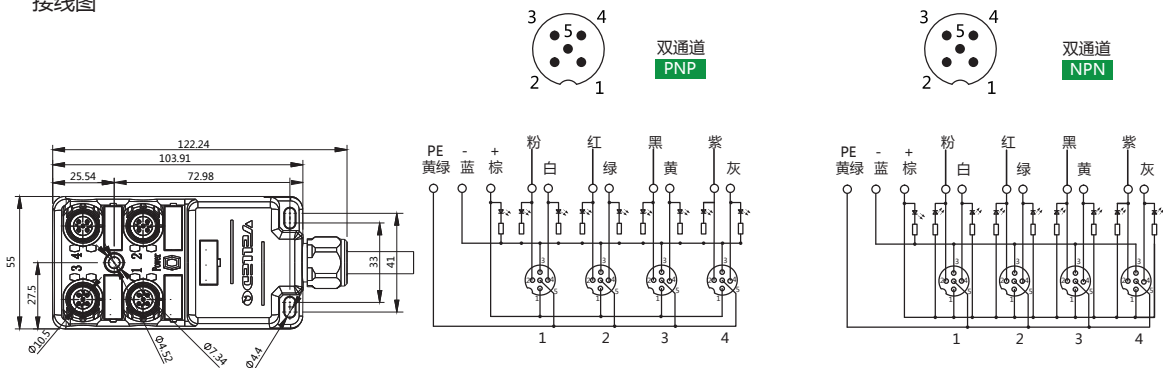
接线图
