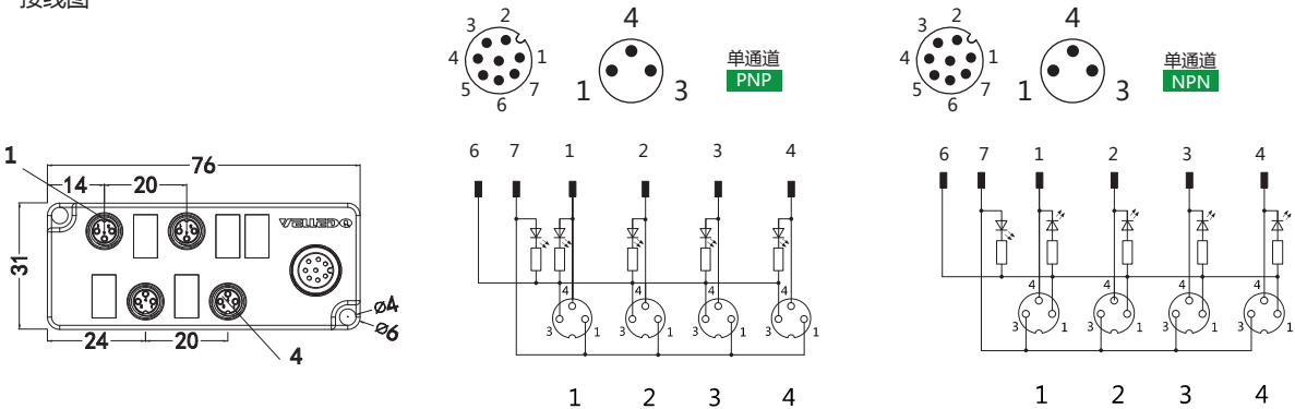
接线图
