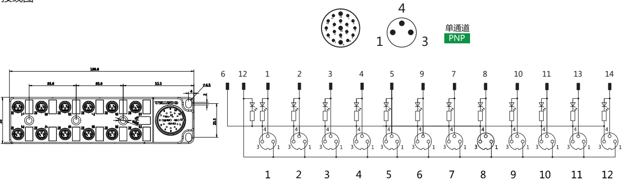
接线图
