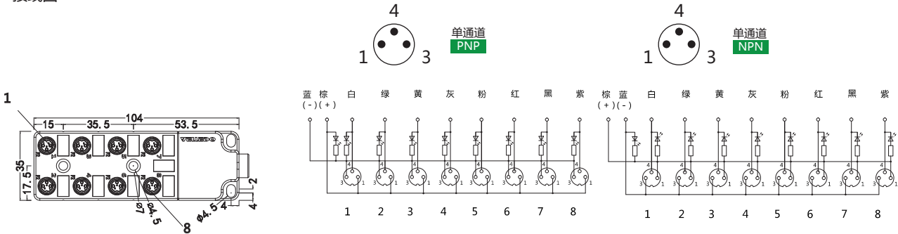
接线图
