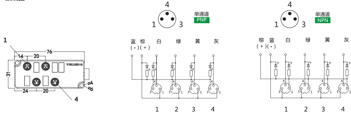
接线图
