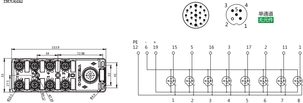
接线图
