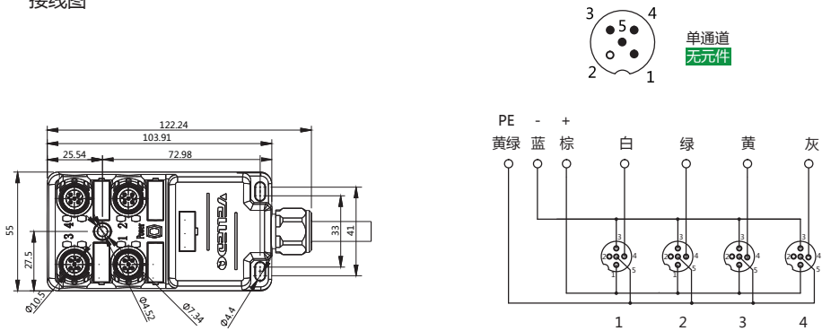
接线图
