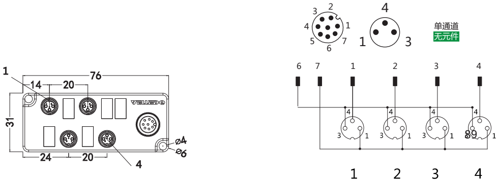
接线图
