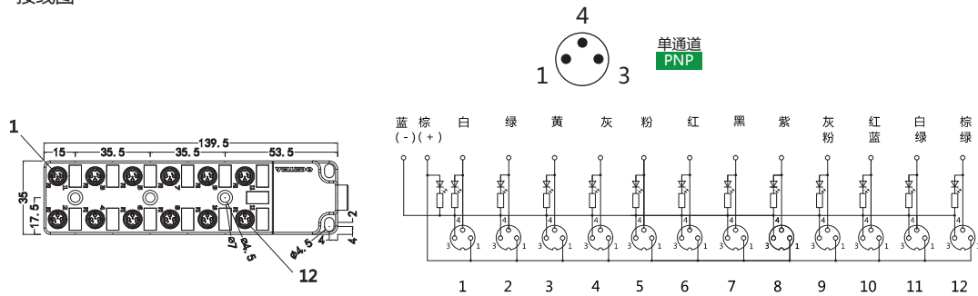
接线图
