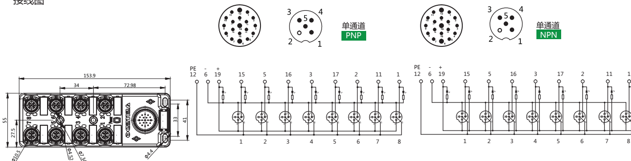
接线图
