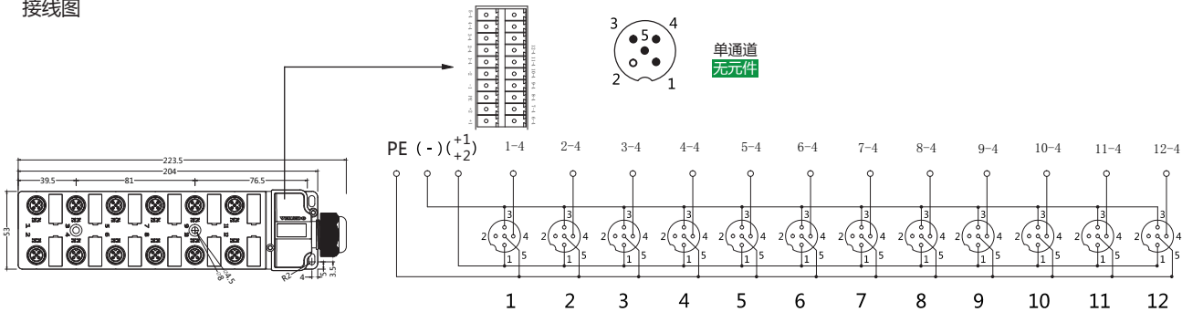
接线图
