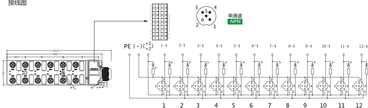
接线图
