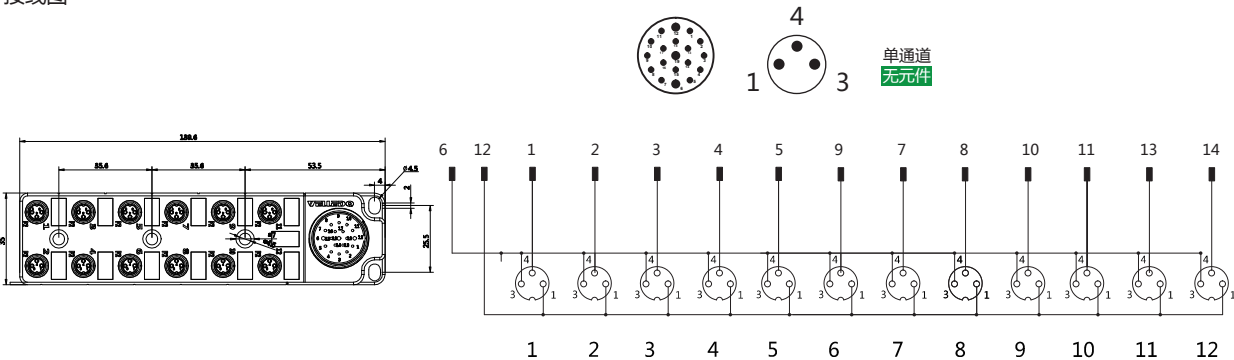
接线图
