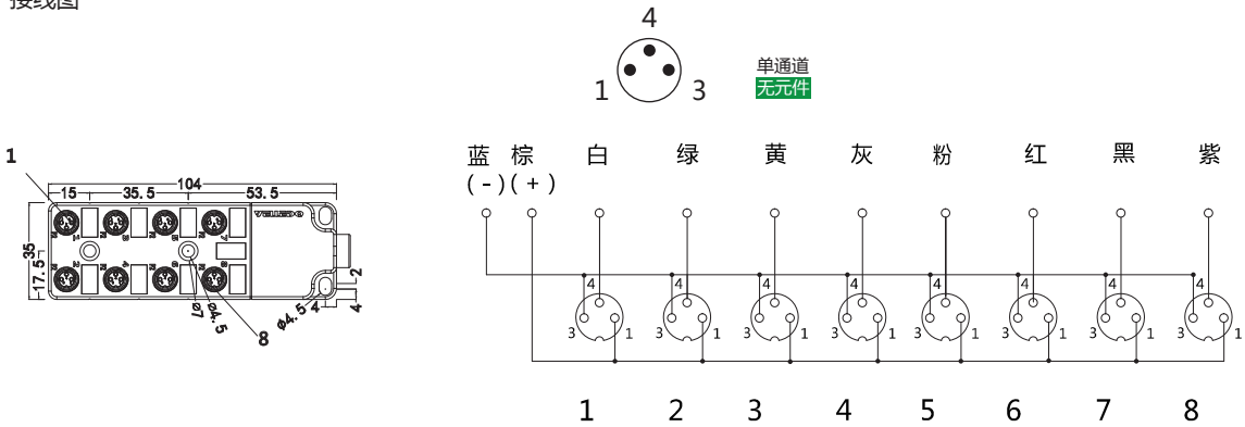
接线图
