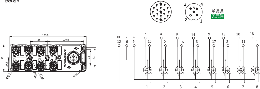
接线图
