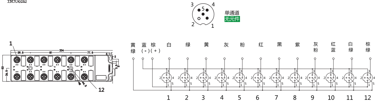
接线图
