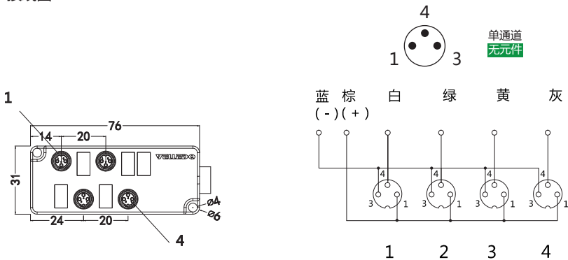
接线图
