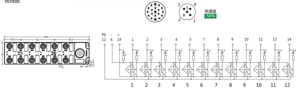
接线图
