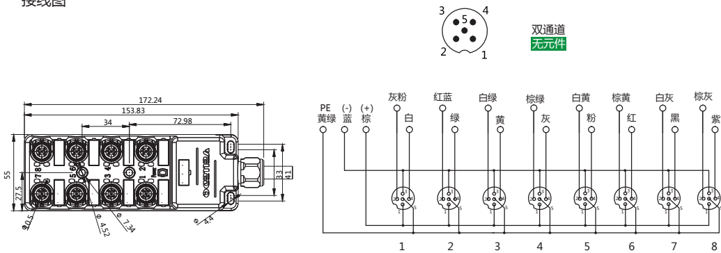
接线图
