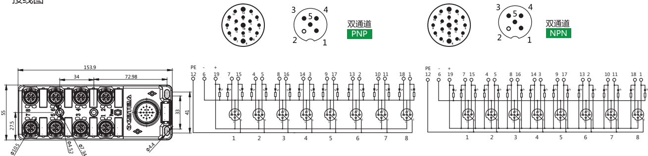
接线图
