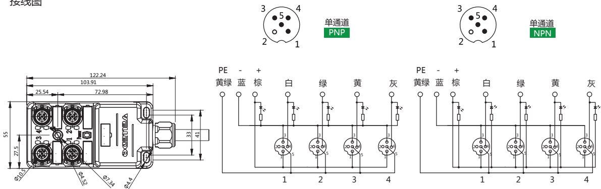
接线图
