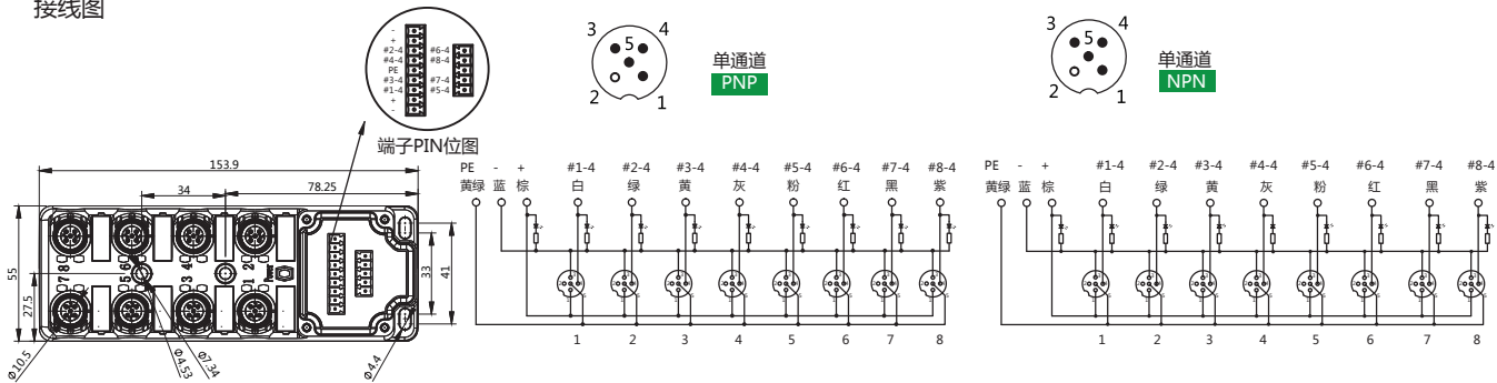
接线图
