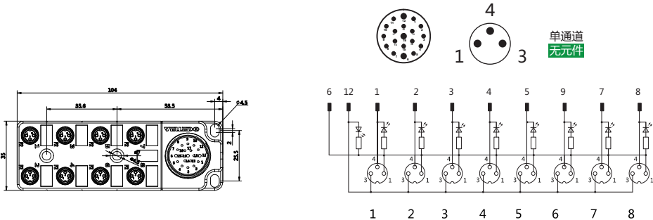
接线图
