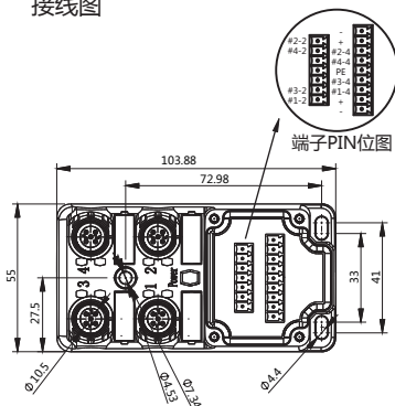
接线图
