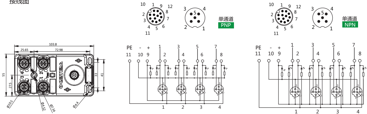
接线图
