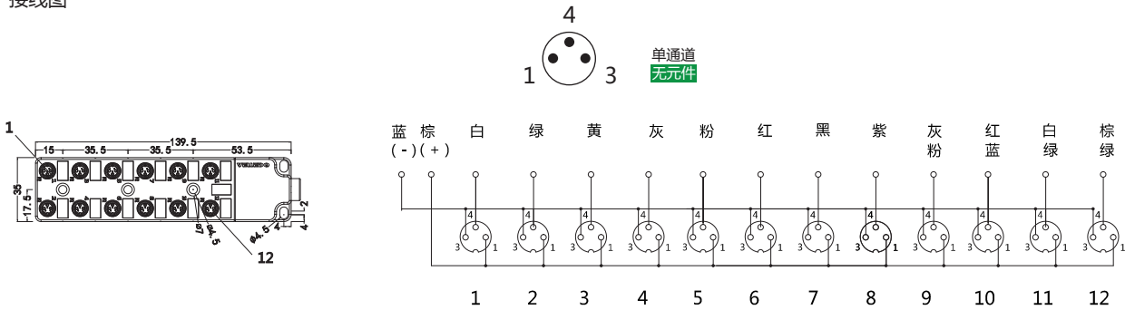
接线图
