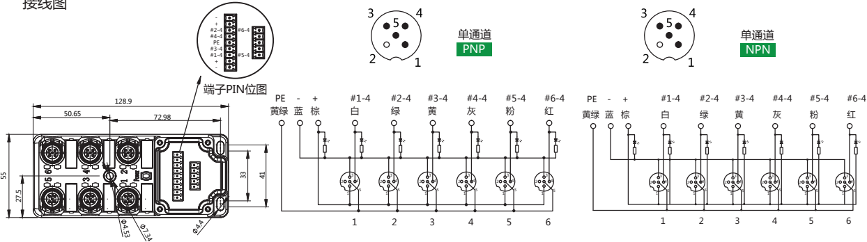
接线图
