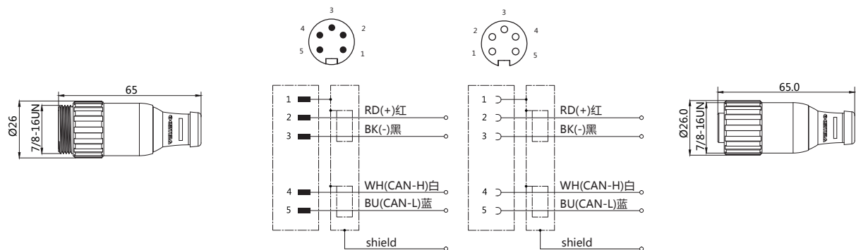
接线图
