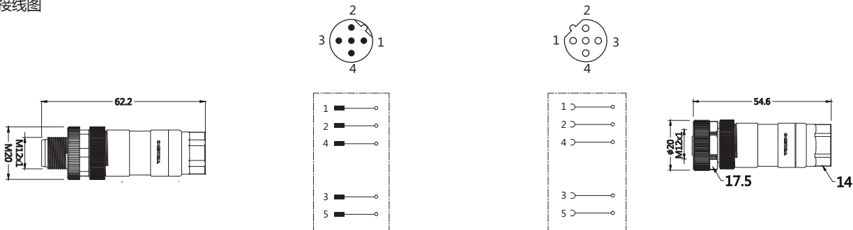
接线图
