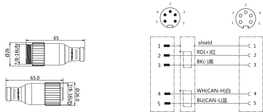
接线图
