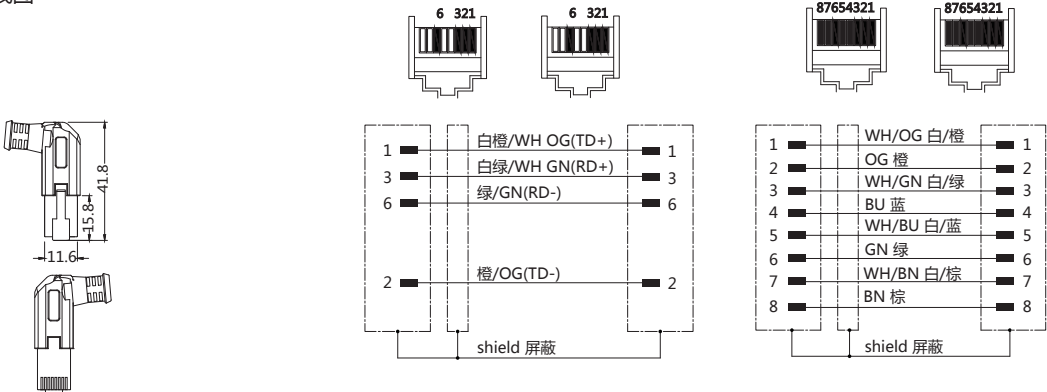
接线图
