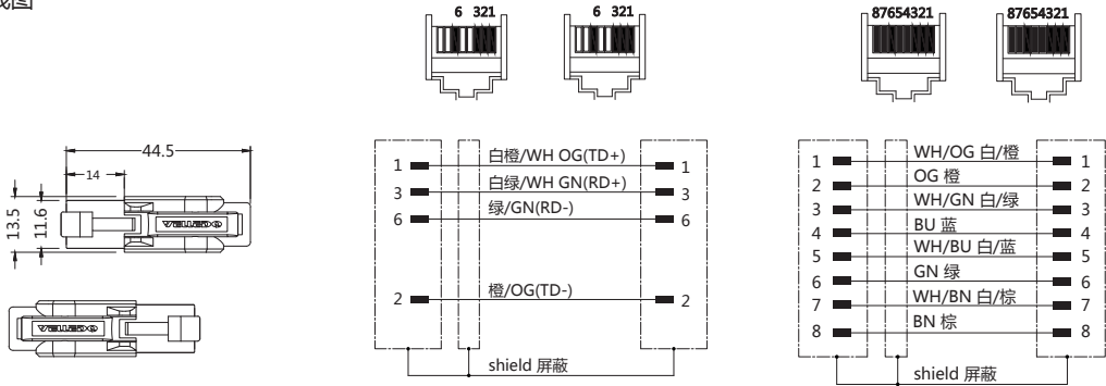
接线图
