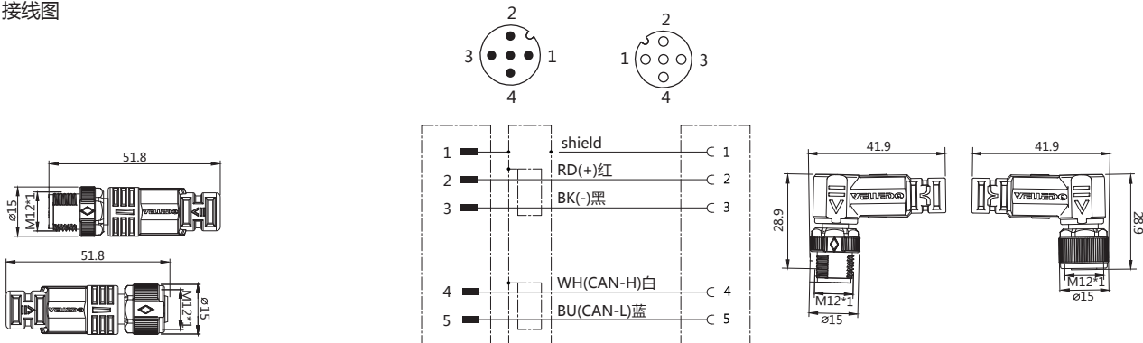
接线图
