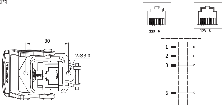
接线图
