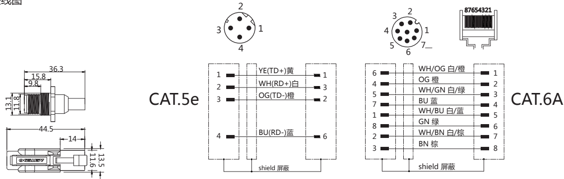
接线图
