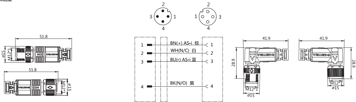
接线图
