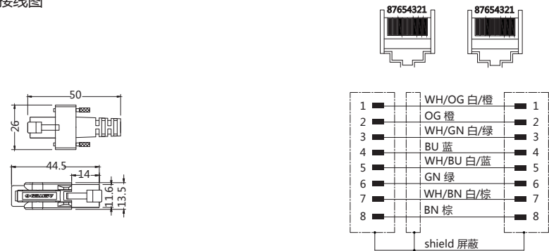
接线图
