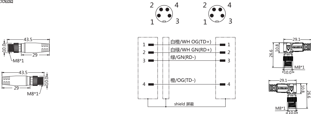
接线图
