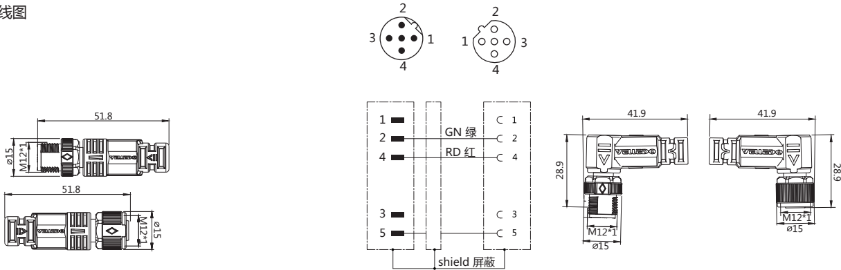
接线图
