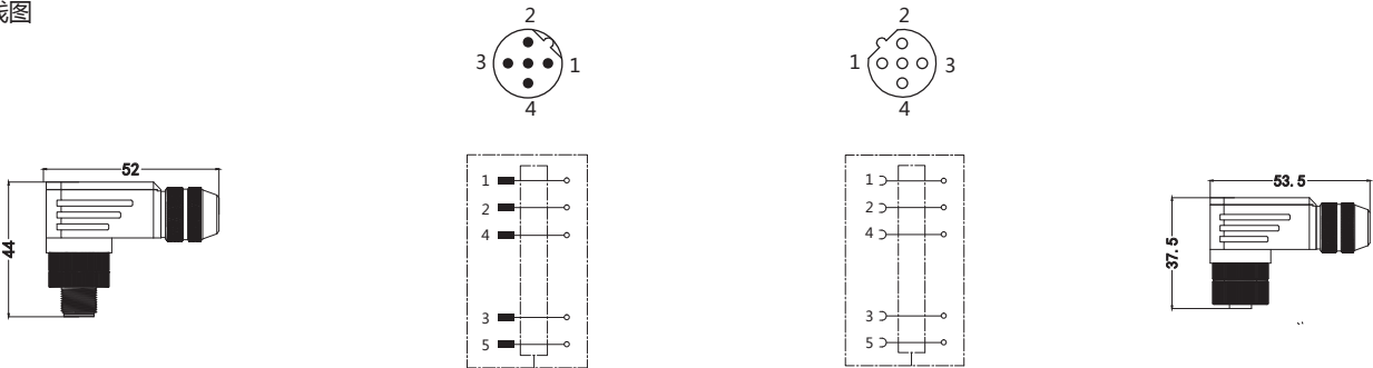
接线图
