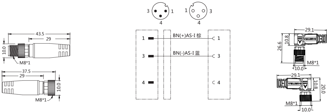
接线图
