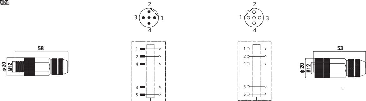
接线图
