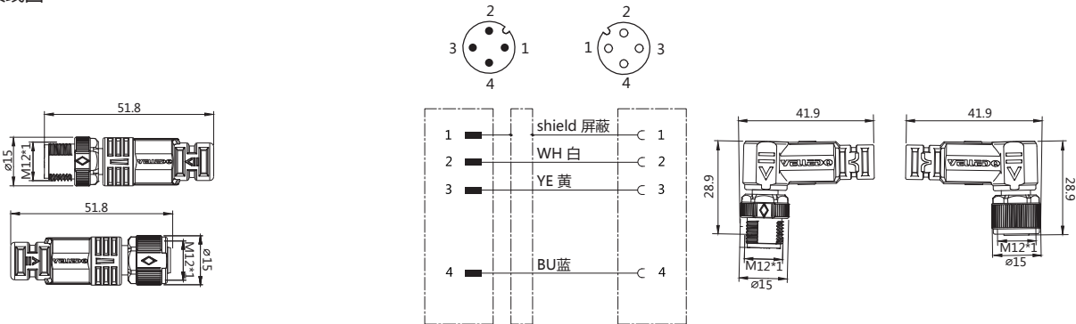
接线图
