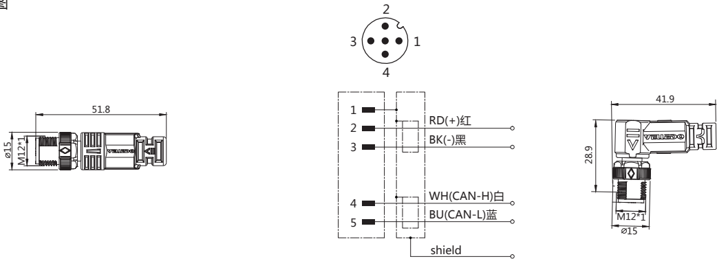
接线图
