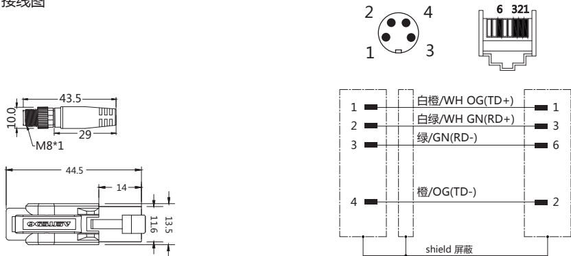
接线图
